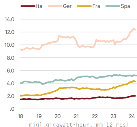
PRODUZIONE DI ENERGIA, IMPIANTI EOLICI
