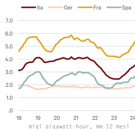
PRODUZIONE DI ENERGIA, IDROELETTRICO
